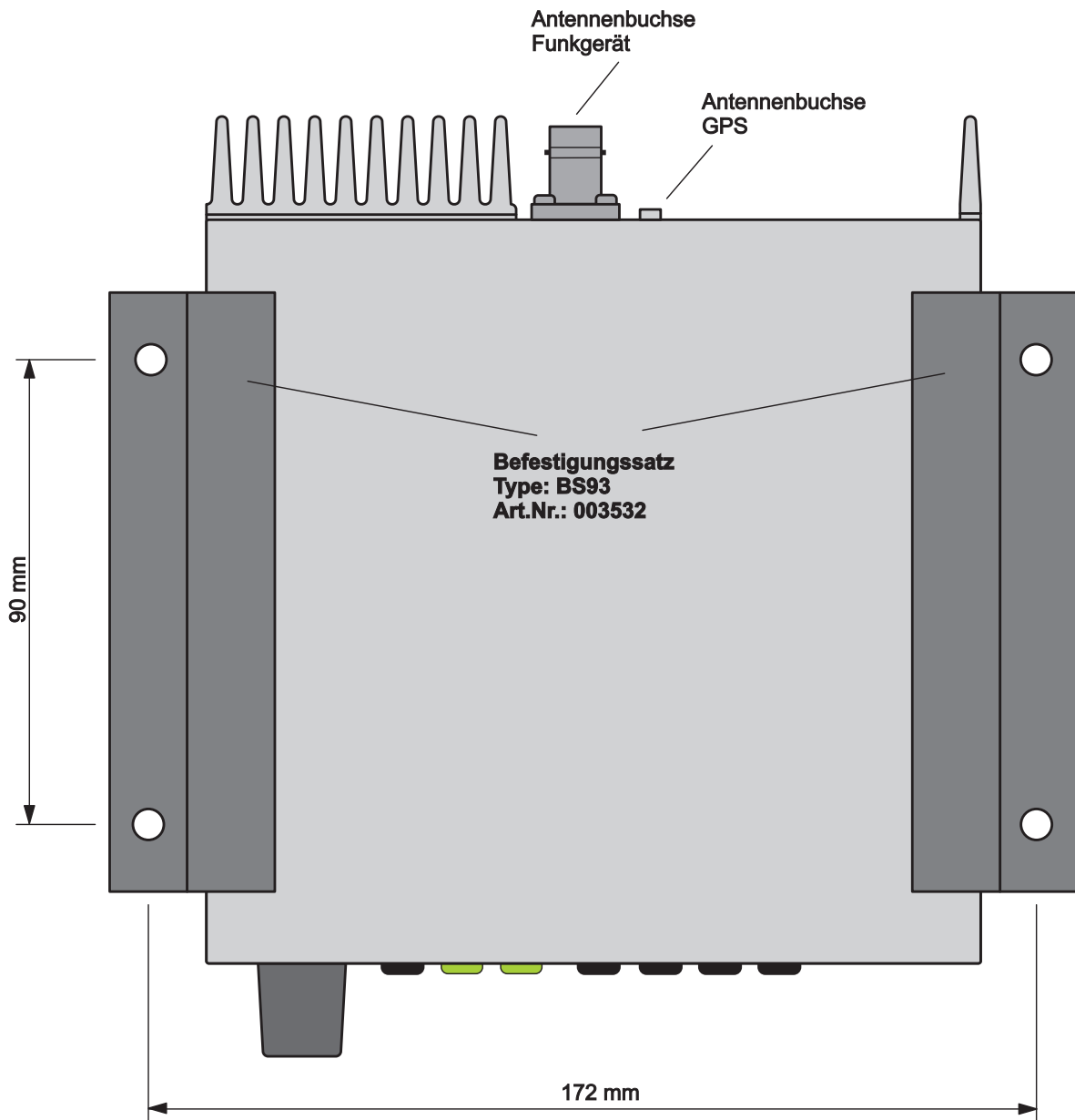
Ansicht: Befestigungssatz BS93 mit Funkgerät M25
