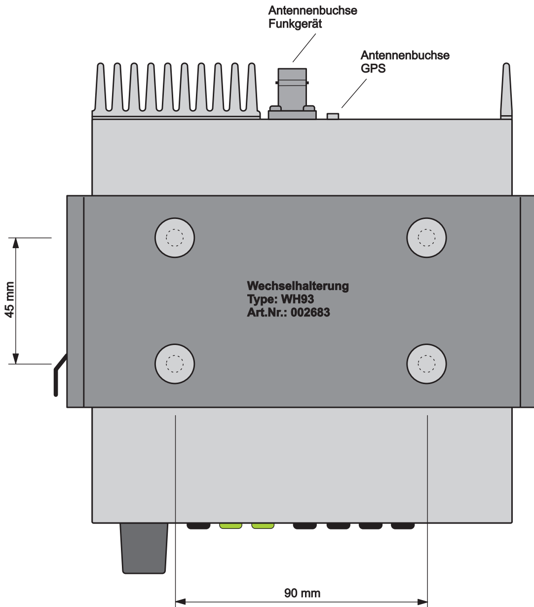
Ansicht: Wechselhalterung WH93 mit Funkgerät M25
