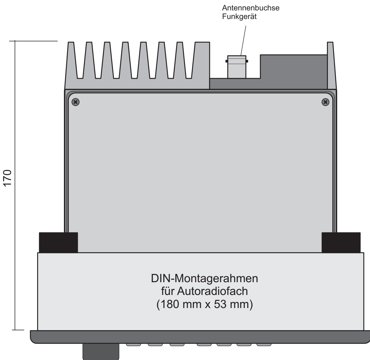
Ansicht: Radiofachhalterung ARH93 mit Funkgerät M93
