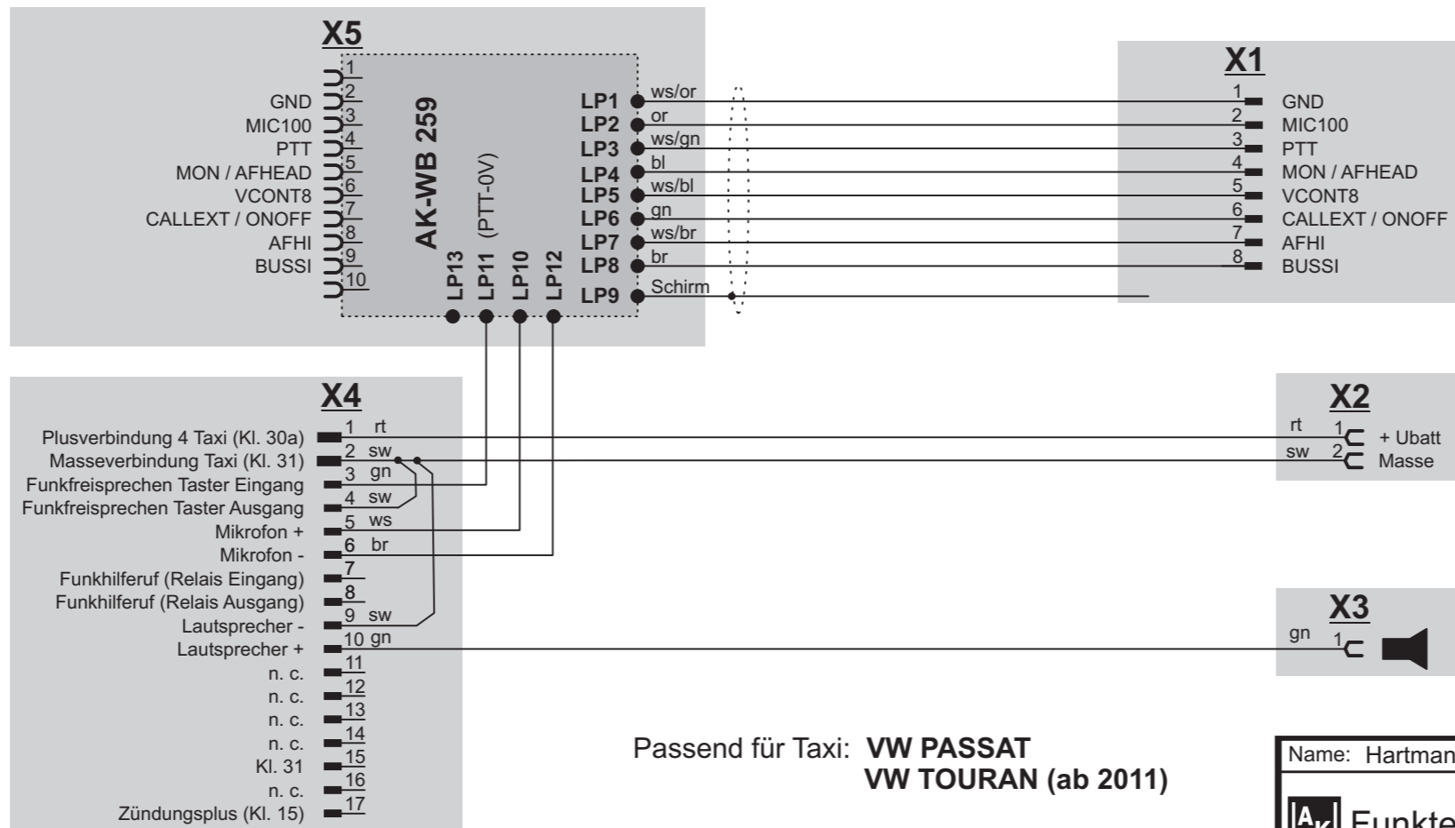
Steckergehäuse zum Anschluß an VW-Stecker 17-polig
