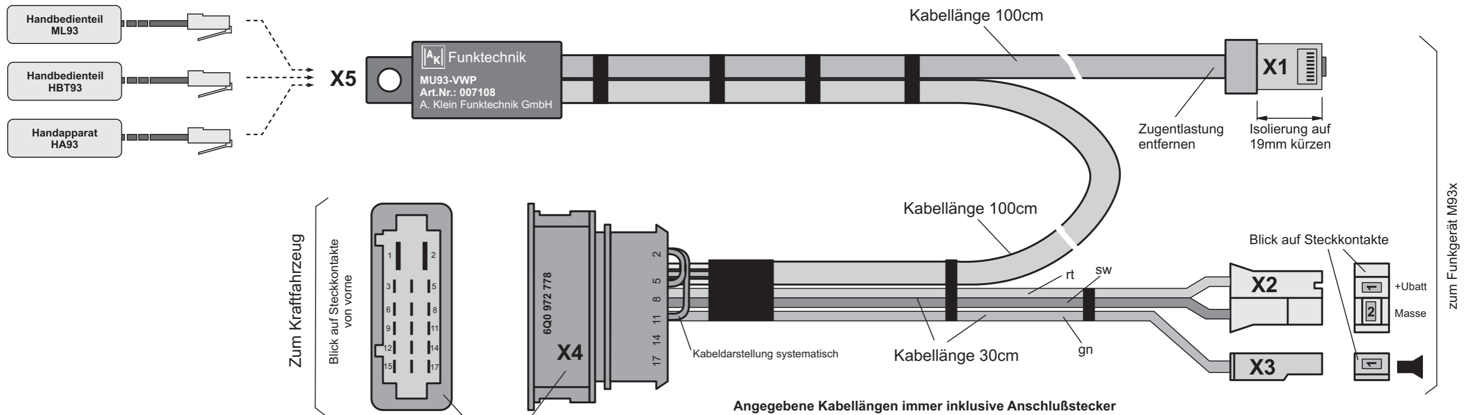
Steckergehäuse zum Anschluß an VW-Stecker 17-polig
