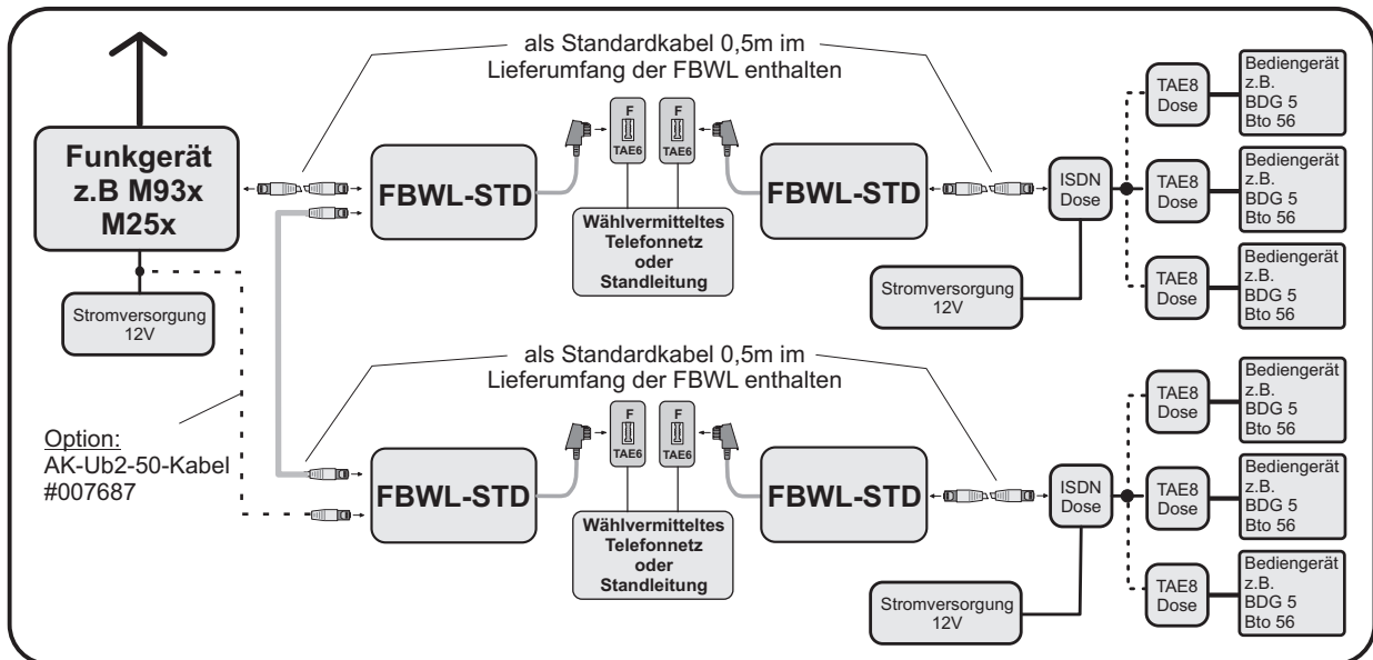
Installationsschema für 2 FBWL-Strecken mit Funkgerät und 2x3 Bediengeräten
